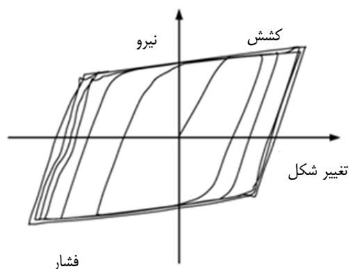
بادبند کماتش ناپذیر
