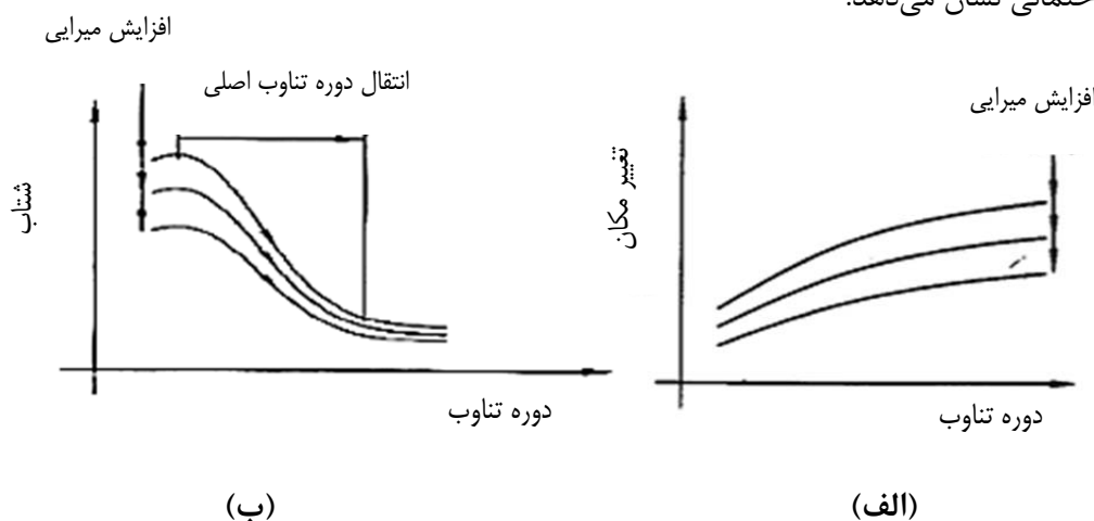
شکل الف-۱- نحوه عملکرد جداساز لرزه ای: (الف) انتقال دوره تناوب اصلی جهت کاهش انرژی وارد، (ب) افزایش میرایی جهت محدود نمودن تغییر مکان (رابینسون ۱۹۹۸)
